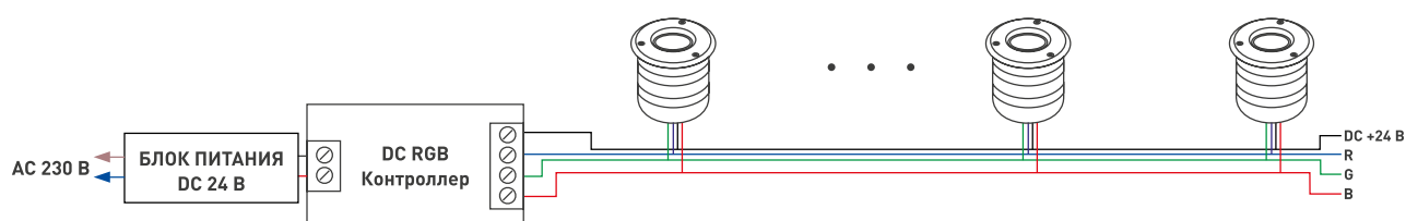
Рис. 3. Схема подключения прожектора к контроллеру RGB
