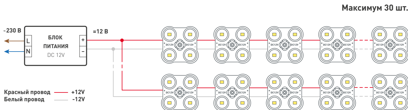
Схема 1. Подключение модулей.
